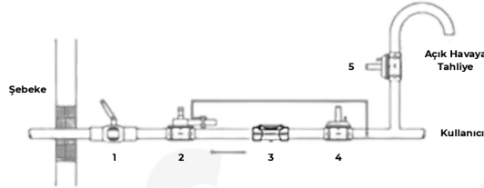
Şekil 1 - Gaz Filtresi Montaj
