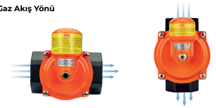
Şekil 2 - Yatay Montaj Yönü
